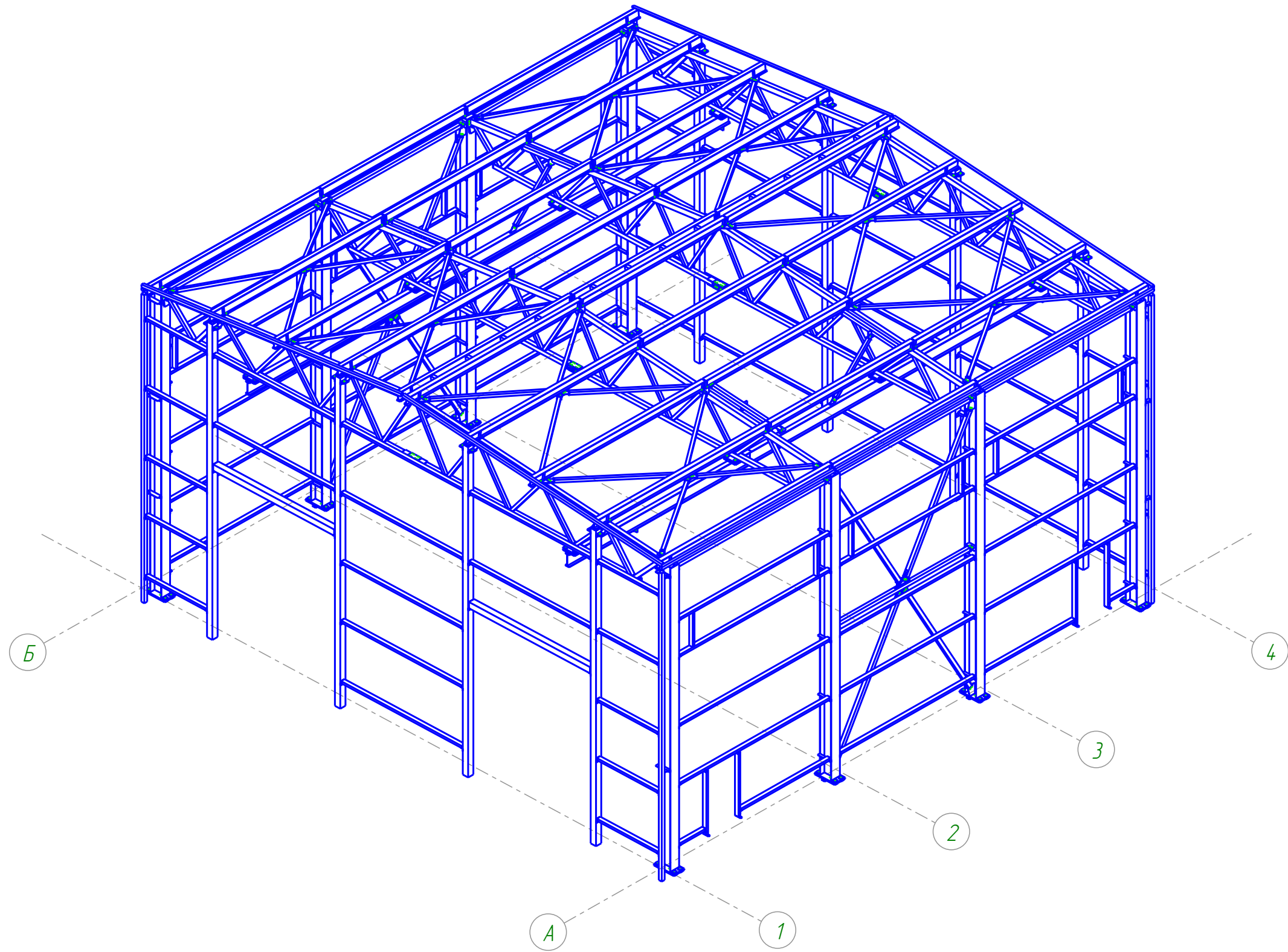
АксонOMETрическая схема каркаса
